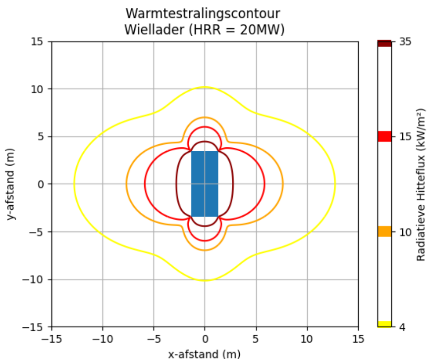
Figuur 9.6 Warmtestralingscontouren wiellader
